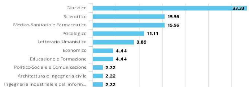
Diplomati nell'a.s.2020/2021 che si sono immatricolati all'università nell'a.a.2021/2022, per gruppi disciplinari (%)
